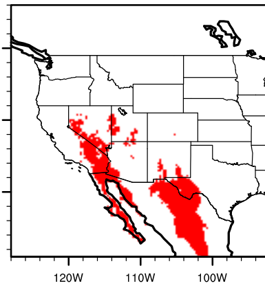
IPSL future yuccfaxo
