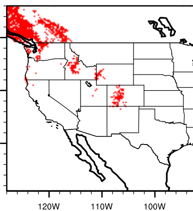
PCM1 future saliscou
