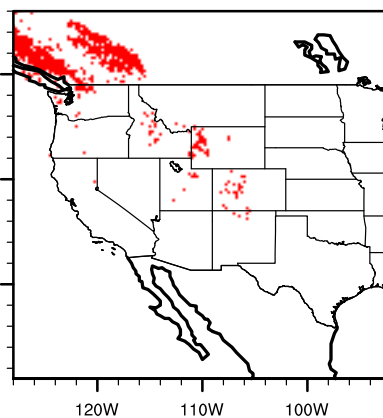
IPSL future saliscou
