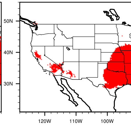
PCM1 future salinigr
