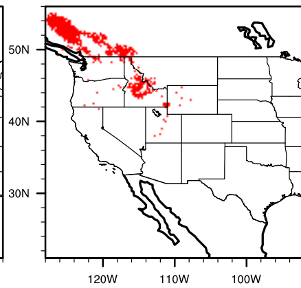
IPSL future saligege
