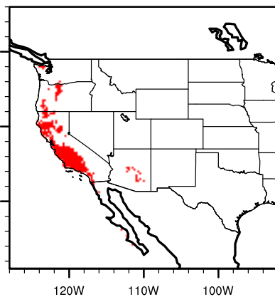
PCM1 future rhamcali
