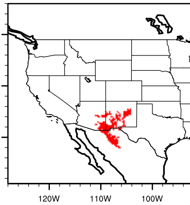
PCM1 future querhypo
