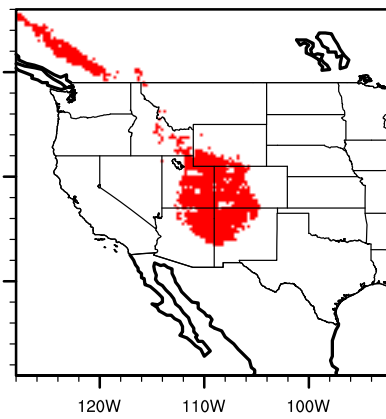
IPSL future quergamb
