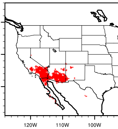
IPSL future querdunn
