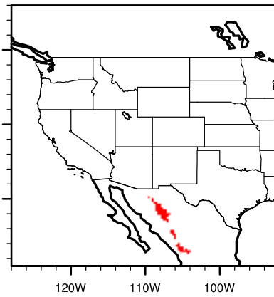
PCM1 future pinudura
