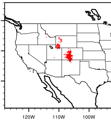
IPSL future picepung
