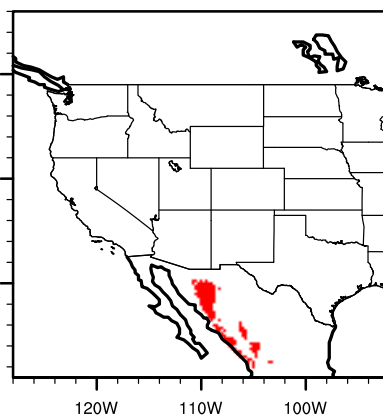
PCM1 future lysimicr
