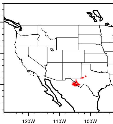
PCM1 future leucretu
