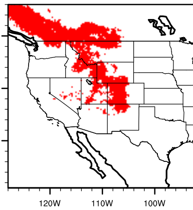
IPSL future juniscop
