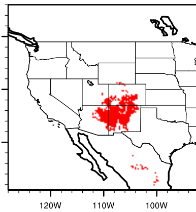
IPSL future junimono
