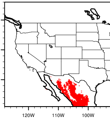
PCM1 future juniflac
