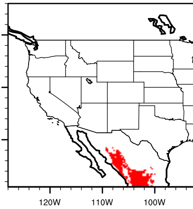
IPSL future juniflac
