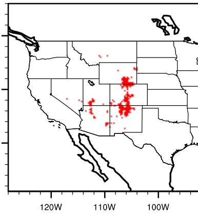
IPSL future junidepp
