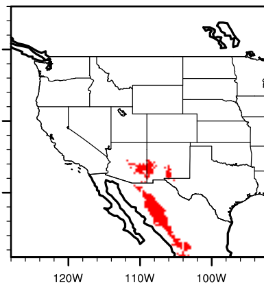
IPSL future juglmajo
