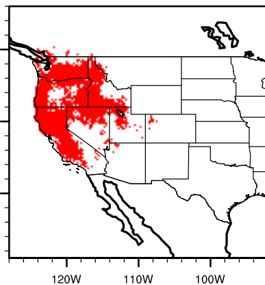
IPSL future fremcali
