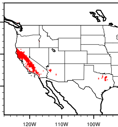
PCM1 future fremcali
