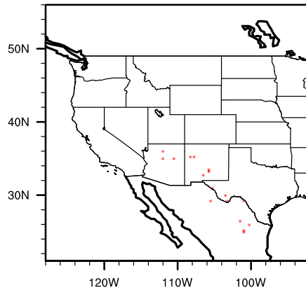
Obs fraxcusp
