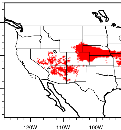
IPSL future celtreti
