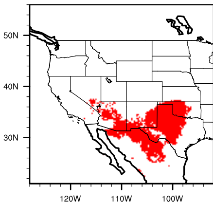
Model modern celtreti
