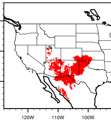
PCM1 future celtreti
