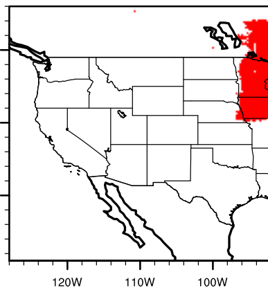
IPSL future celtocci
